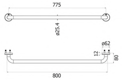
FBVHC-TS790E unit : mm
